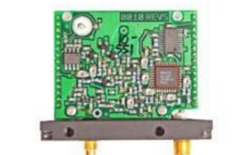
Module permettant la transmission par ondes radio
